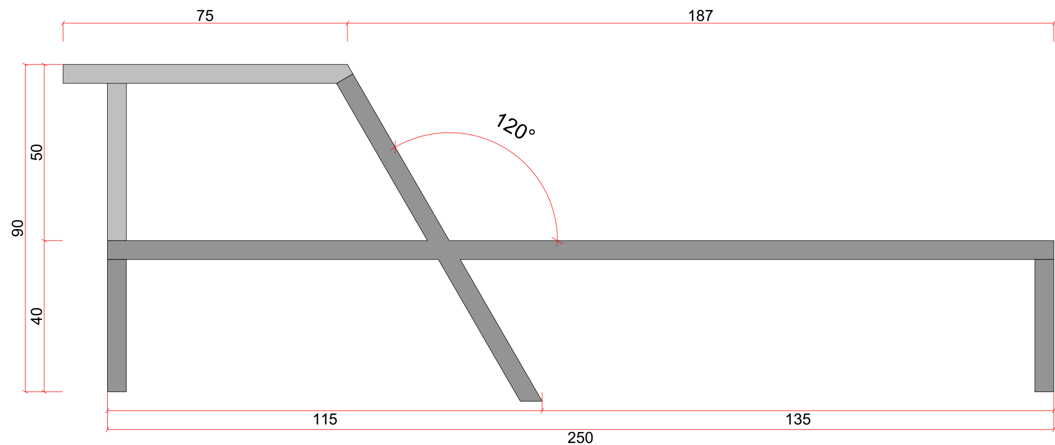
VISTA LAT. DIREITA ESC: 1/10
