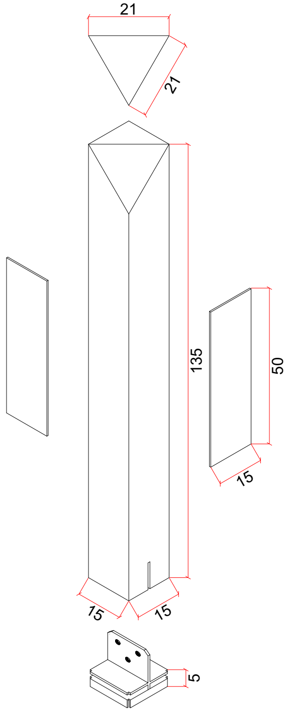
ISOMÉTRICA EXPLODIDA ESC: 1/10
