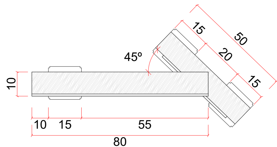
VISTA FRONTAL ESC: 1/10
