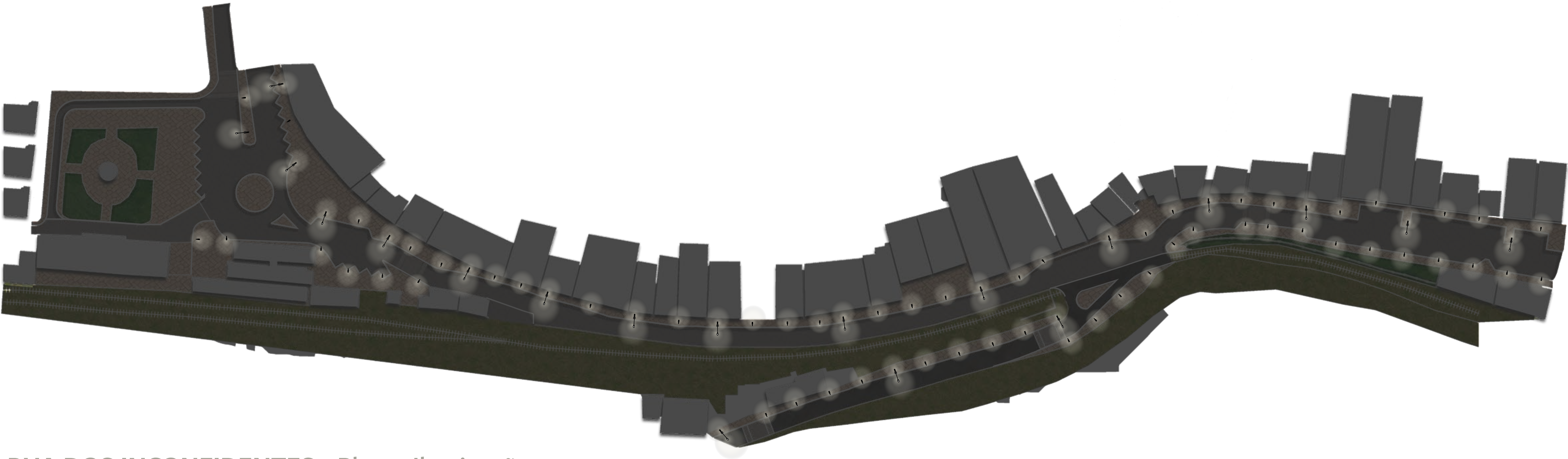
RUA DOS INCONFIDENTES - Planta Iluminação ESCALA 1:750
