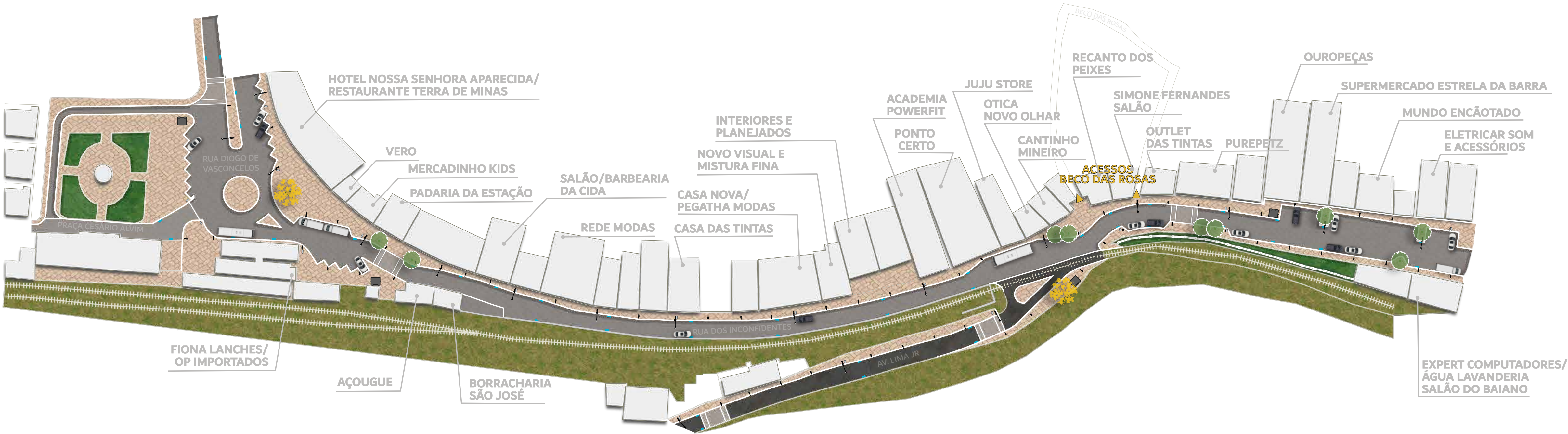
RUA DOS INCONFIDENTES - Planta Humanizada ESCALA 1:750
