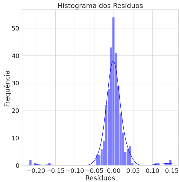
Figura 9 – Histograma dos resíduos.
