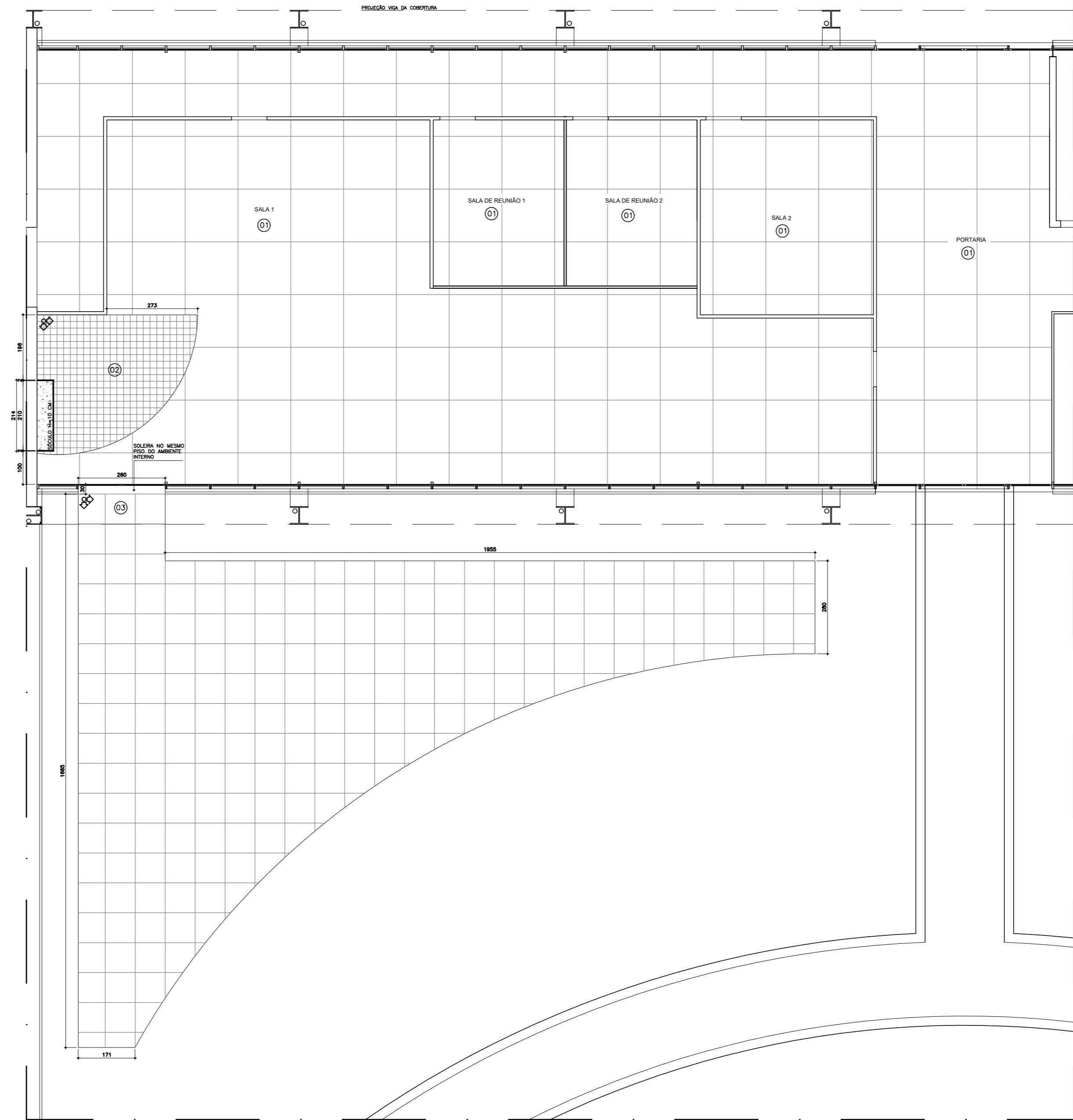
PAVIMENTO TÉRREO PLANTA PISOS ESC 1/100
