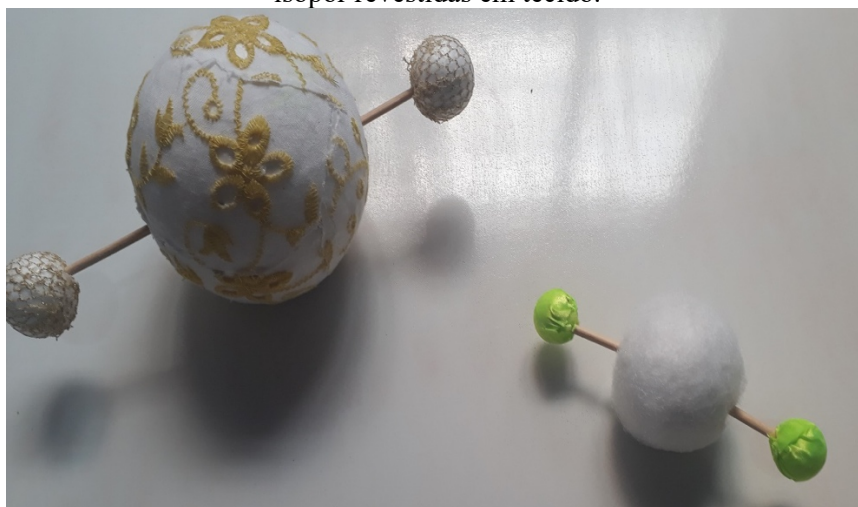
Figura 17: Representação da geometria molecular linear, utilizando palitos de madeira e bolinhas de isopor revestidas em tecido.
