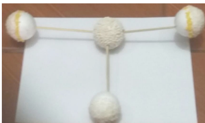
Figura 5 - Representação da Geometria molecular Trigonal Plana Triflureto de Boro ( \text{BF}_3 ).
