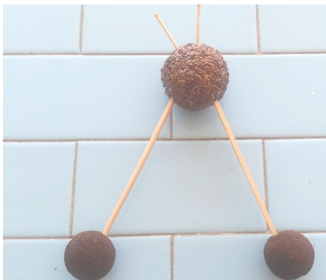
Figura 4- Representação da Geometria molecular angular da água ( \text{H}_2\text{O} ).
