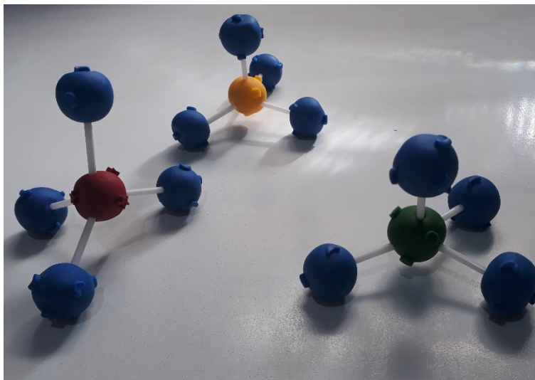
Figura 22: Representação da geometria molecular tetraédrica, utilizando bolinhas confeccionadas com massa de biscoito e palitos plásticos
