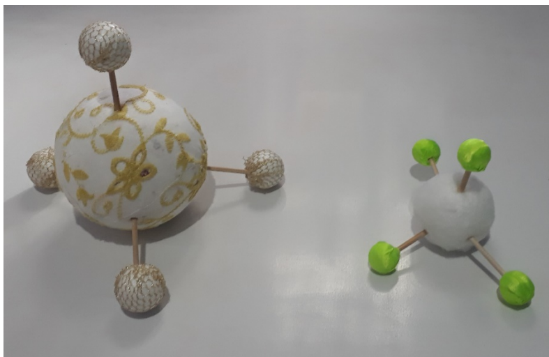
Figura 23: Representação da geometria molecular tetraédrica, utilizando palitos de madeira e bolinhas de isopor revestidas em tecido
