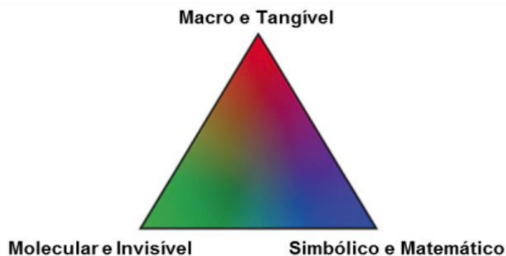
Figura: 1 - Modelo de Johnstone para os níveis de representação do conhecimento químico
